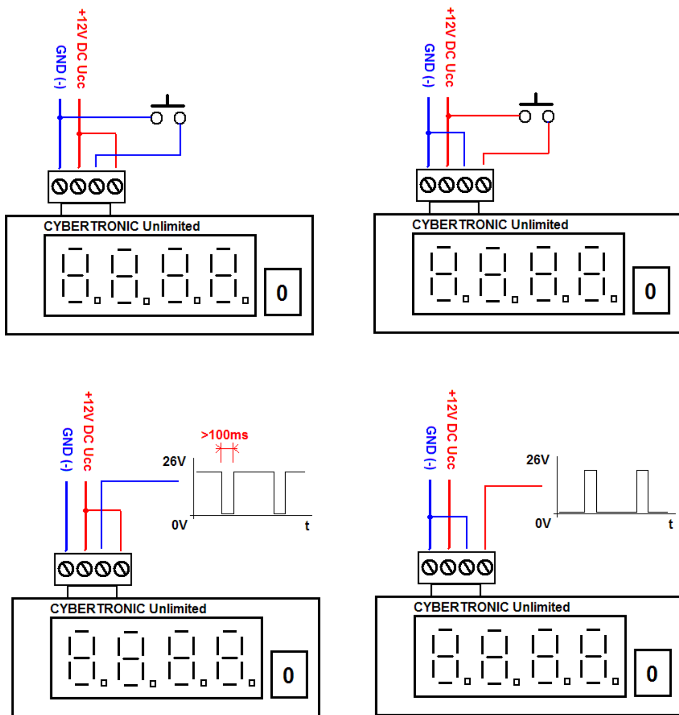
Obrázek 2.: Způsob zapojení počítačla CLC Kit
