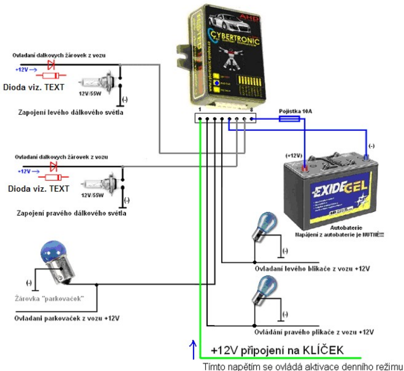
Obrázek 1. Schéma zapojení
