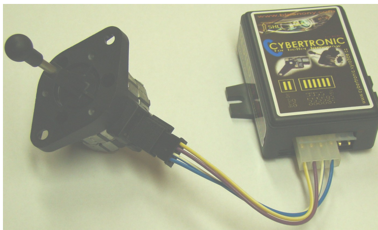
Obrázek 2. SHL komplet se zapojením
