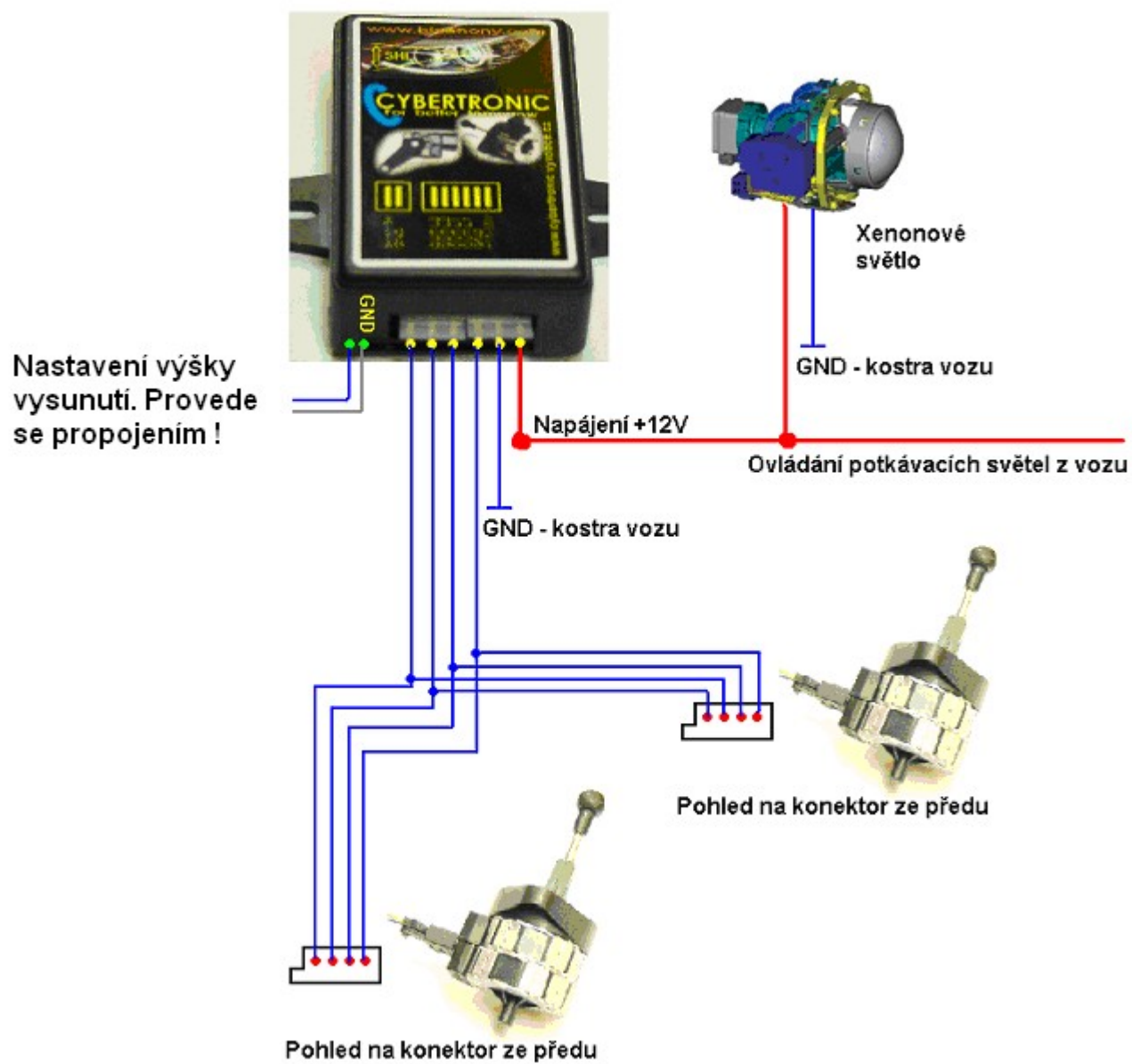
Obrázek 6. Schéma zapojení
