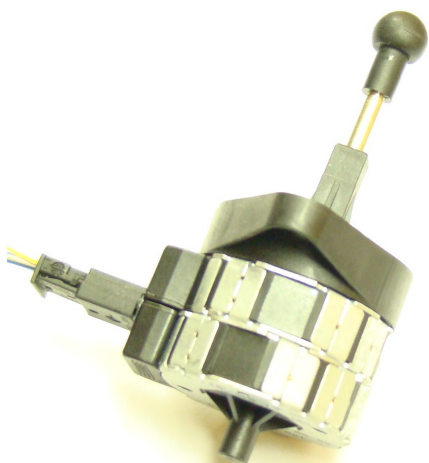
Obrázek 1. 4-drátový krokový motor
